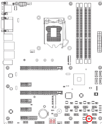
JP13 → COM2 Header
