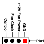
CPUFAN
